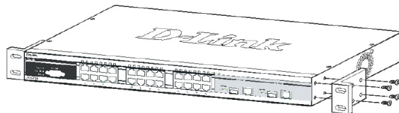
图2. 安装机架挂耳
