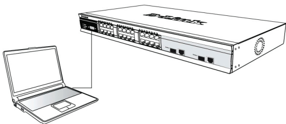
图 9. 通过配置线缆连接PC
