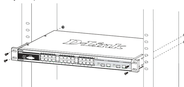
Рисунок 3. Установка коммутатора
