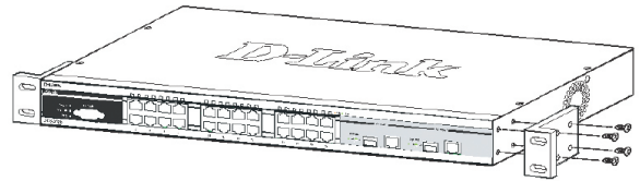
圖 2. 裝上固定架
