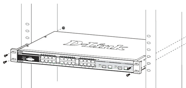
Figure 3. Installation du switch dans une armoire de taille standard
