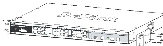
Figura 2. Fijación de los ángulos de montaje
