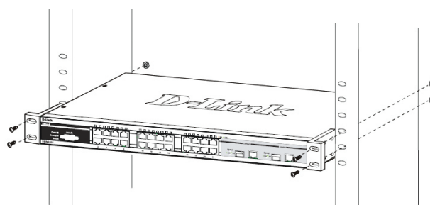
図3 スイッチをラックに取り付ける
