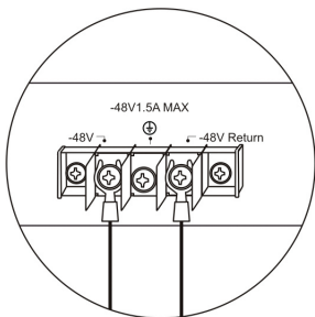
图 5. 将电源接点连接到电源组的触点上
