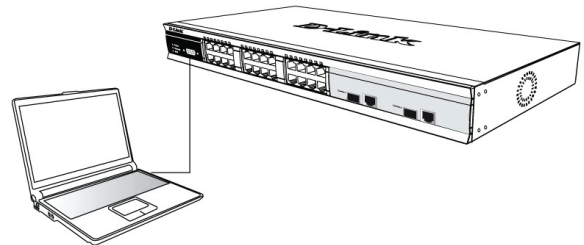
Abbildung 9. Endgerät verbunden über ein Konsolenkabel
