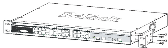
Abbildung 2. Befestigung der Rack-Einbauwinkel
