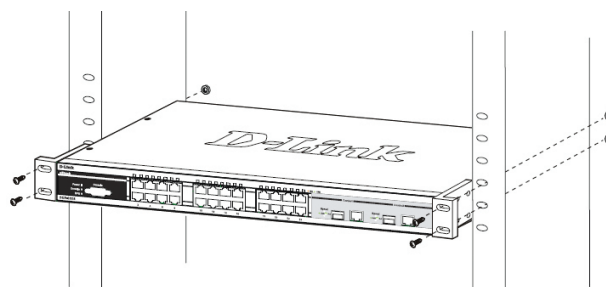
Figura 3. Instalación del Switch en un rack de tamaño estándar equipment rack
