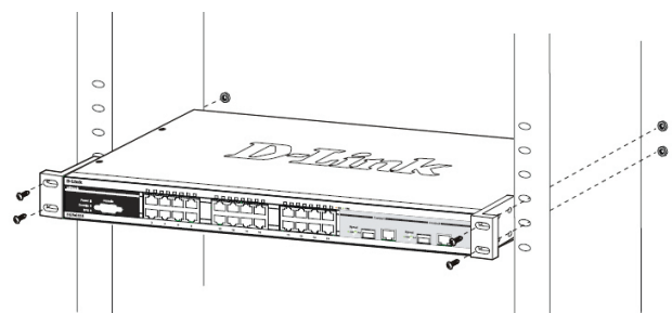
Abbildung 3. Einbau im Standard 19-Zoll Rack
