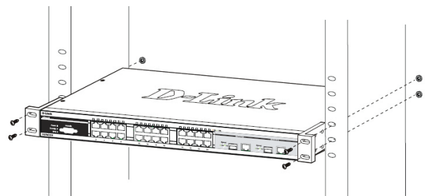
Gambar 3. Memasang switch ke rak dengan ukuran standar
